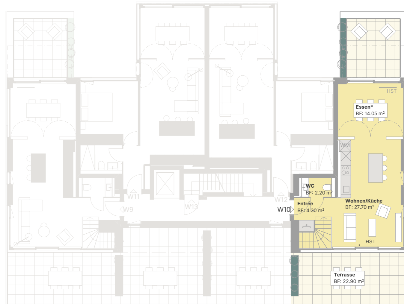
Obergeschoss
